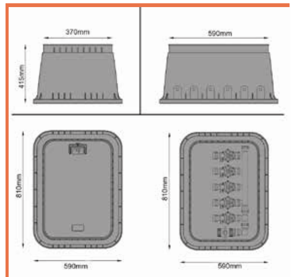
Support de vanne programmeur
